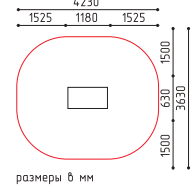
30-006 1180x630x1850 (ДШВ в мм)
