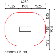
30-004 1180x500x1850 (ДШВ в мм)
