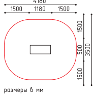
30-007 1180x630x1850 (ДШВ в мм)
